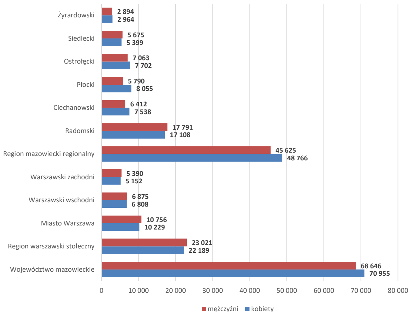
Wykres 2. Liczba osób bezrobotnych wg płci w podregionach województwa mazowieckiego
