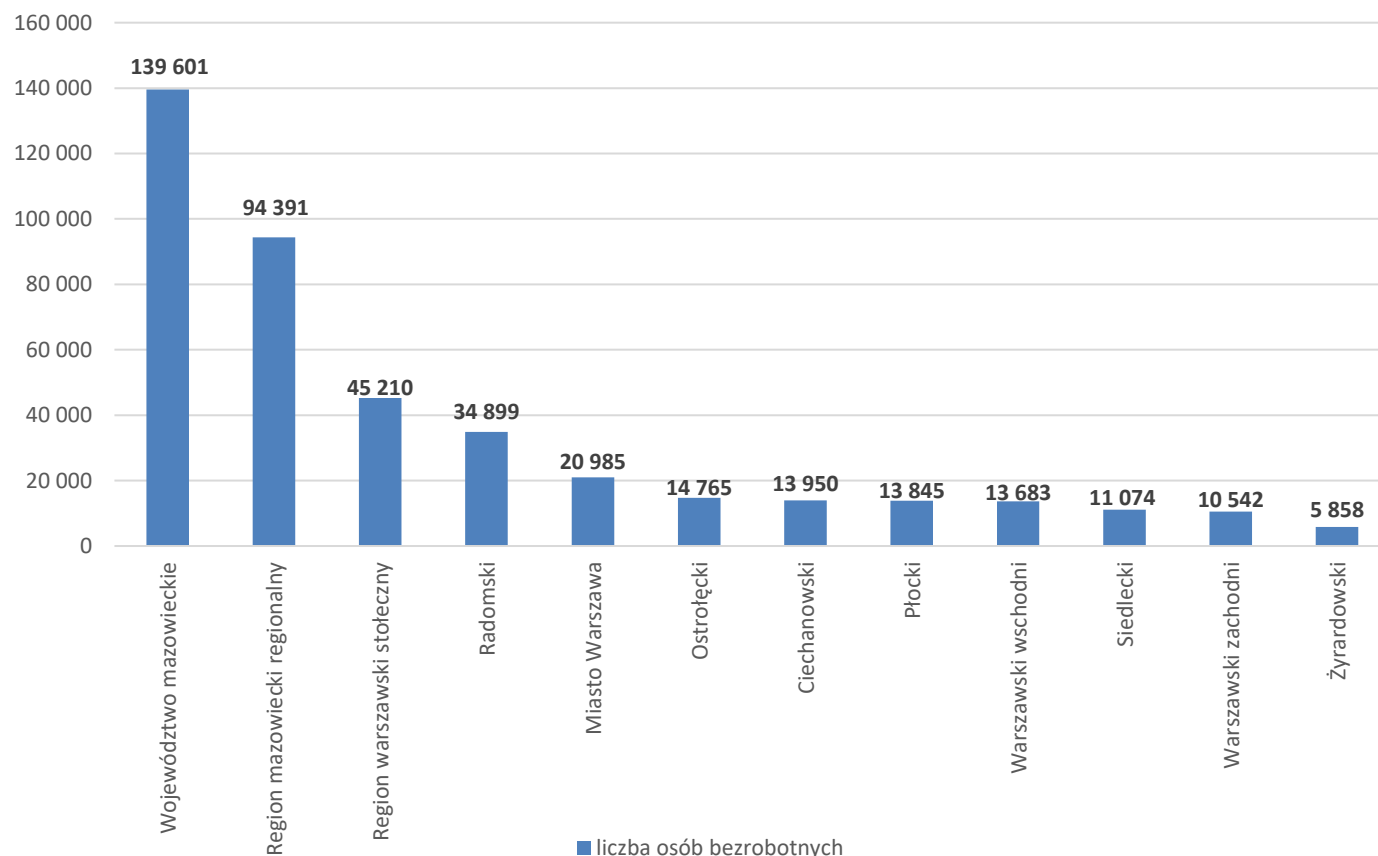
Wykres 1. Liczba osób bezrobotnych w podregionach województwa mazowieckiego
